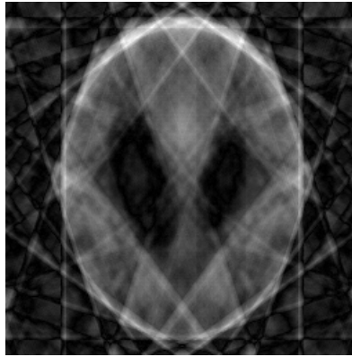
\text{vec}^{-1} f
